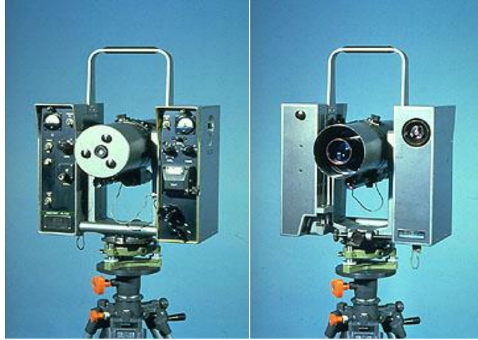
الشكل 5.7: جهاز القياس الكهروضوئي متوسط المدى (10 كم إلى 25 كم) – Geodimeter 6A [14].
