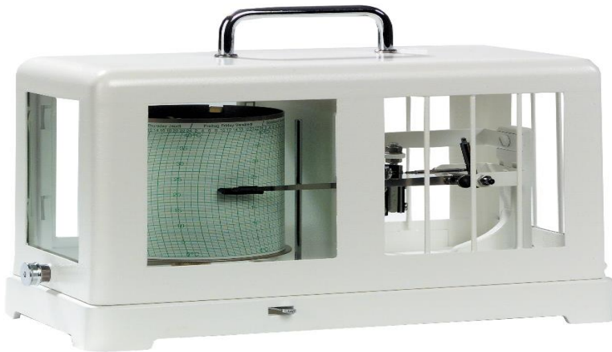
المحرار المسجل Thermograph
