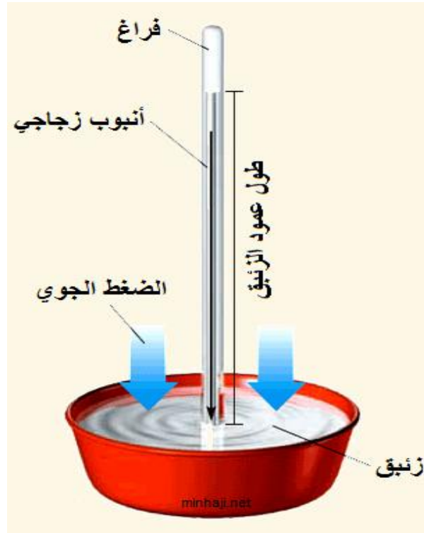
المرواز الزئبقي
