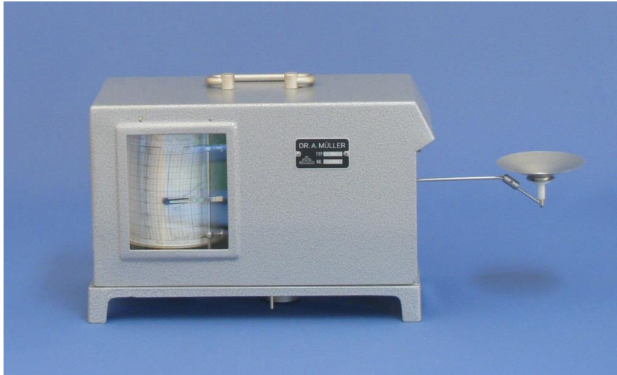
مسجل الندى
