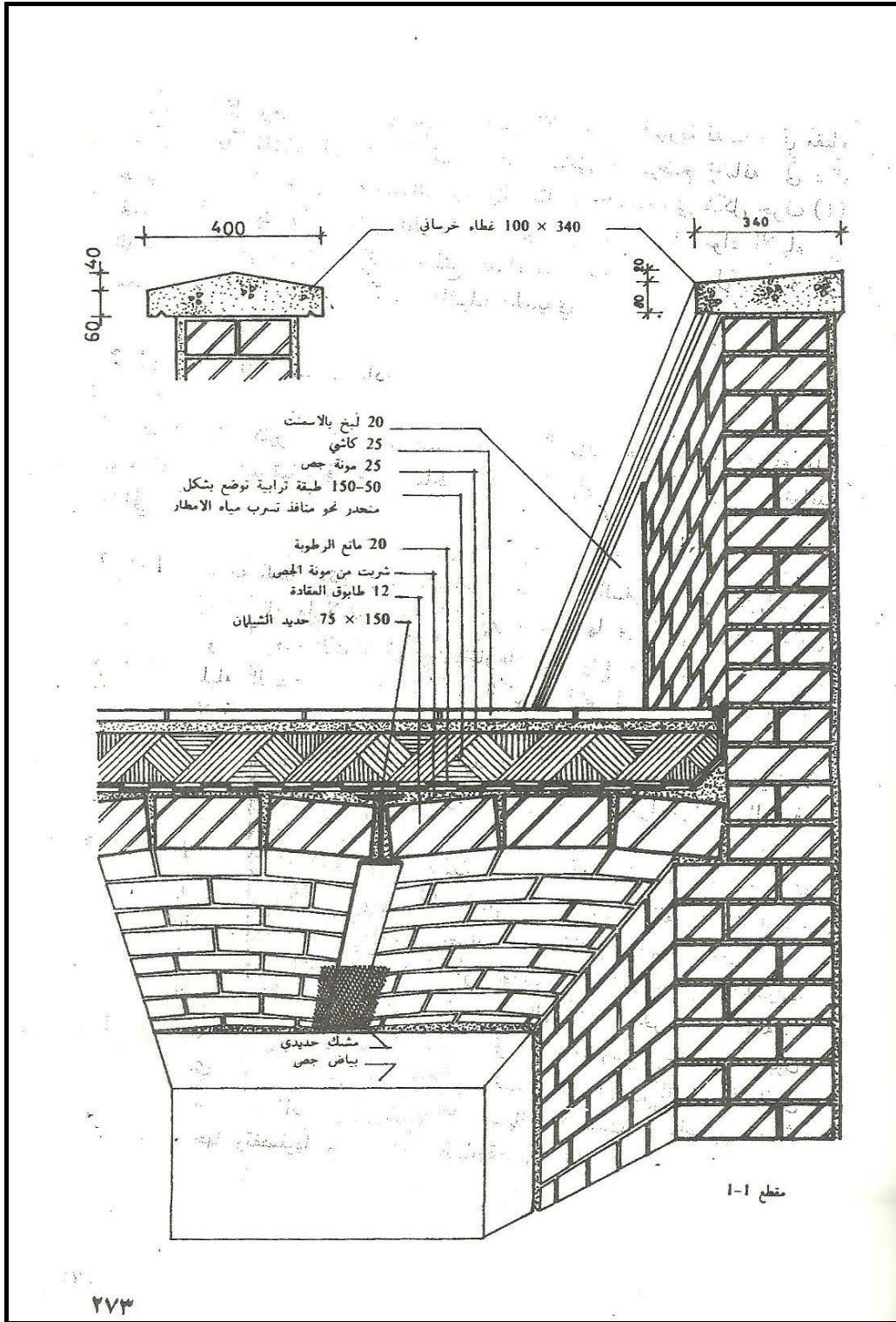
الشكل رقم (٣) التفاصيل الانشائية لسقوف العقادة
