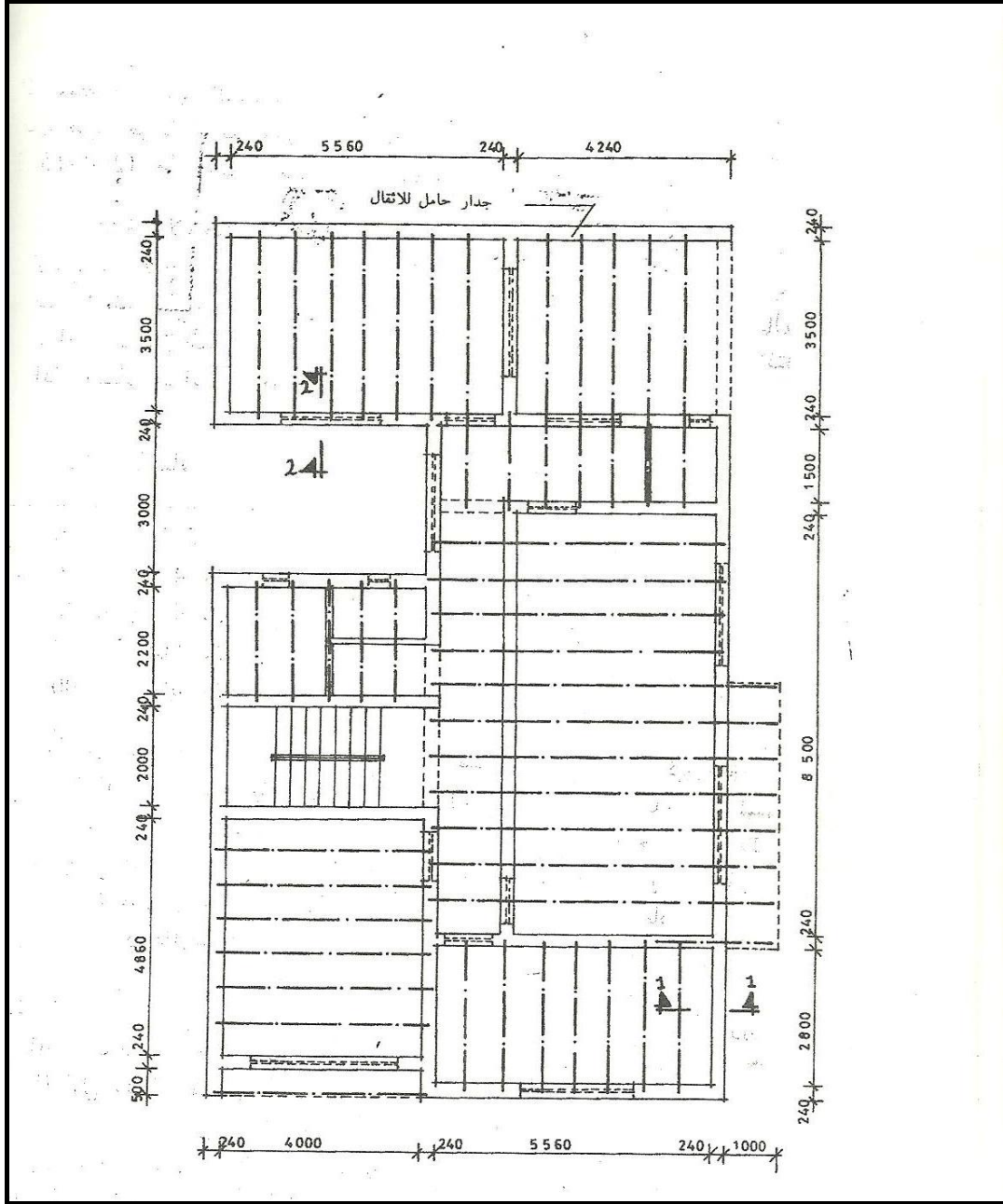
الشكل رقم (1) مخطط افقي يبين توزيع حديد الشيلمان فوق الجدران الحاملة
