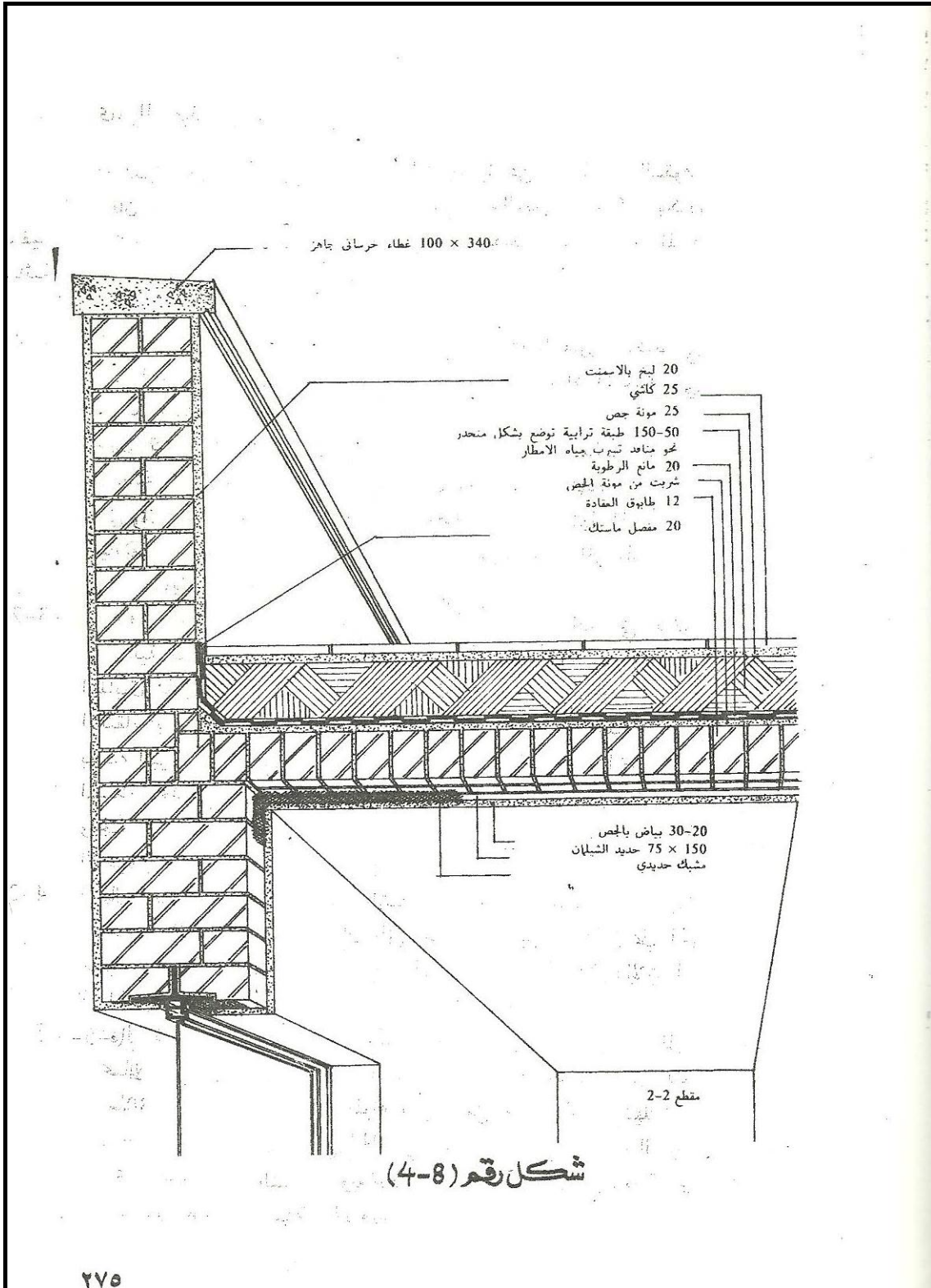
الشكل رقم (٤) مقطع في العقادة باتجاه طول حديد الشيلمان
