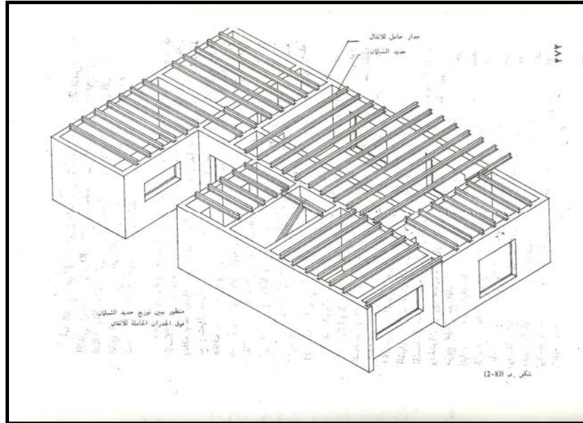
الشكل رقم (٢) توزيع حديد الشيلمان حسب المسافات المقبولة انشائيا
