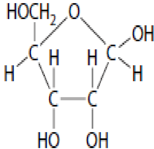
سكر الرايبوز
