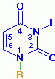
Uracil
