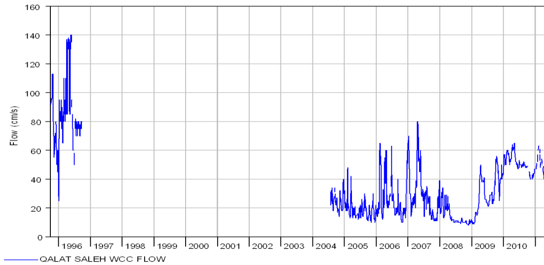
الشكل ١٠ : تصريف نهر دجلة لسنوات مختلفة ( وزارة الموارد المائية/العراق، ٢٠١١م).
