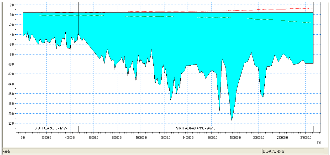
الشكل ٥: المقطع الطولي لشط العرب
