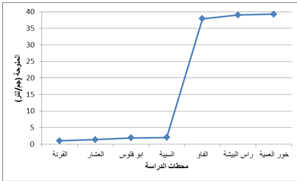
شكل ٩ : التوزيع الطولي للملوحة في محطات مصب شط العرب لشهر يونيو ٢٠١٢م.
