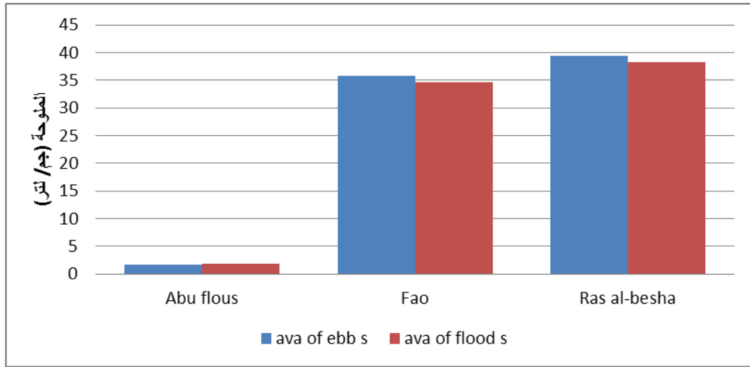
الشكل ١٢: معدل الملوحة لحالتي المد والجزر في مصب شط العرب في محطات (أبو فلوس ، الفاو ، رأس البيشة).
