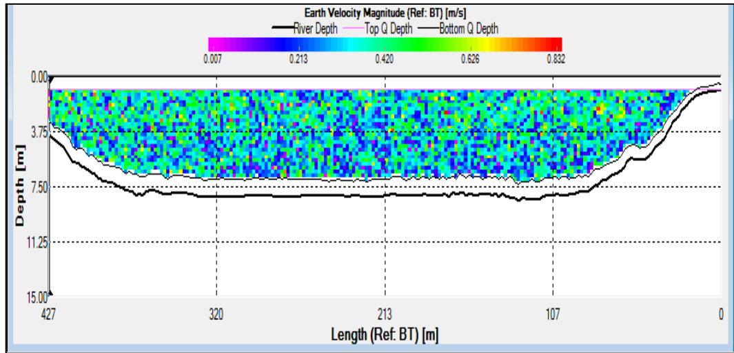
شكل رقم ٣: مقطع عرضي لشط العرب في منطقة القرنة
