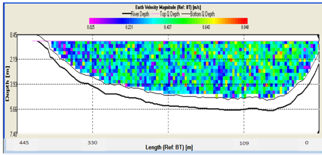
الشكل رقم ٤: مقطع عرضي لشط العرب (مقابل ميناء أبو فلوس)
