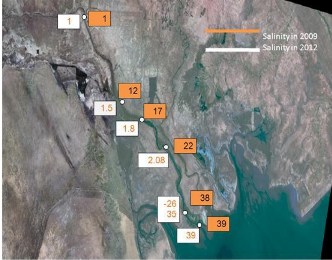
الشكل ١١ : نمط الانتقال الطولي للملوحة في مصب شط العرب حسب هذه الدراسة.
