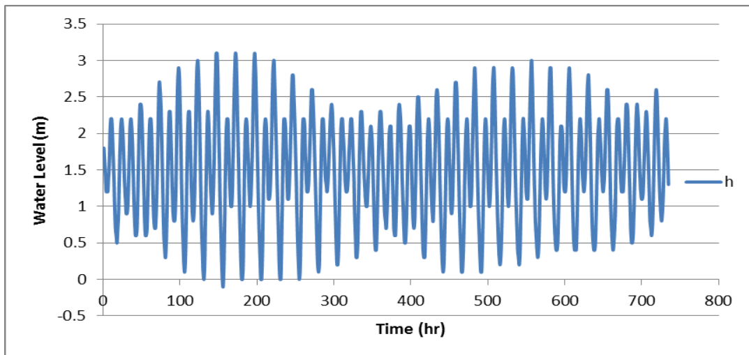
شكل رقم ٢: موجة المد و الجزر في شط العرب
