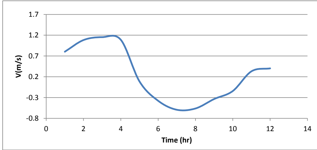
الشكل ٧: سرعة التيار في محطة رأس البيشة ليوم 22/6/2012
