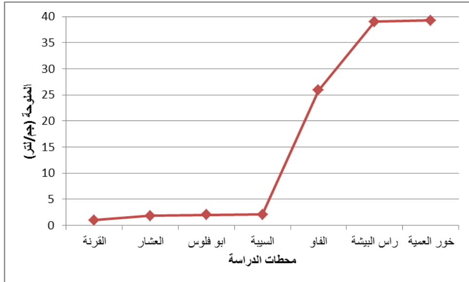
شكل ٨ : التوزيع الطولي للملوحة في محطات مصب شط العرب لشهر مايو ٢٠١٢م.
