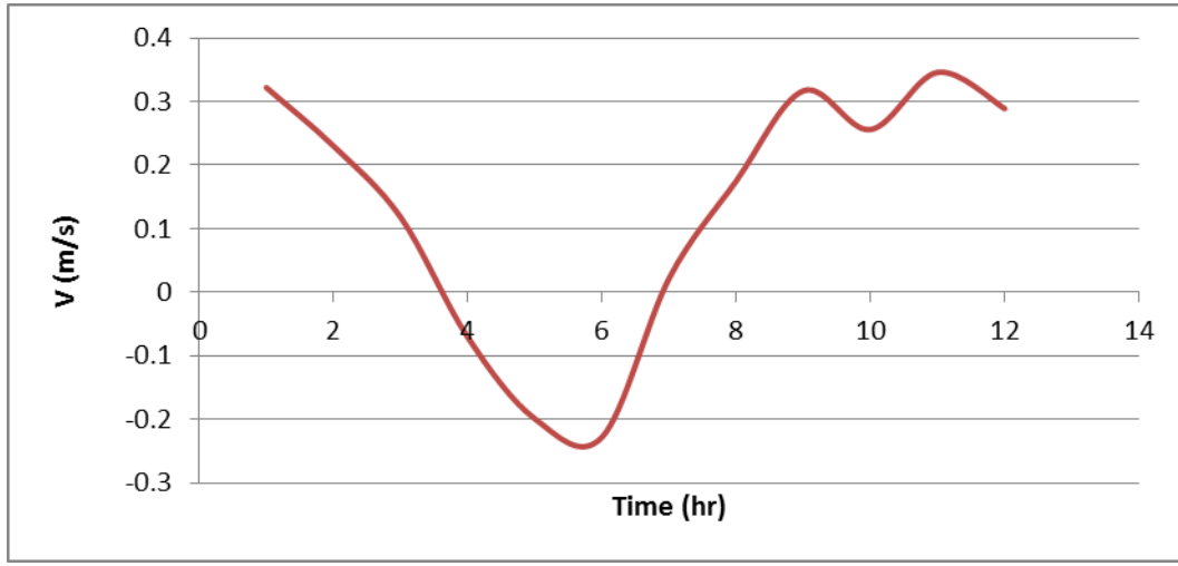
الشكل ٦: سرعة التيار في محطة القرنة ليوم 29/5/2012
