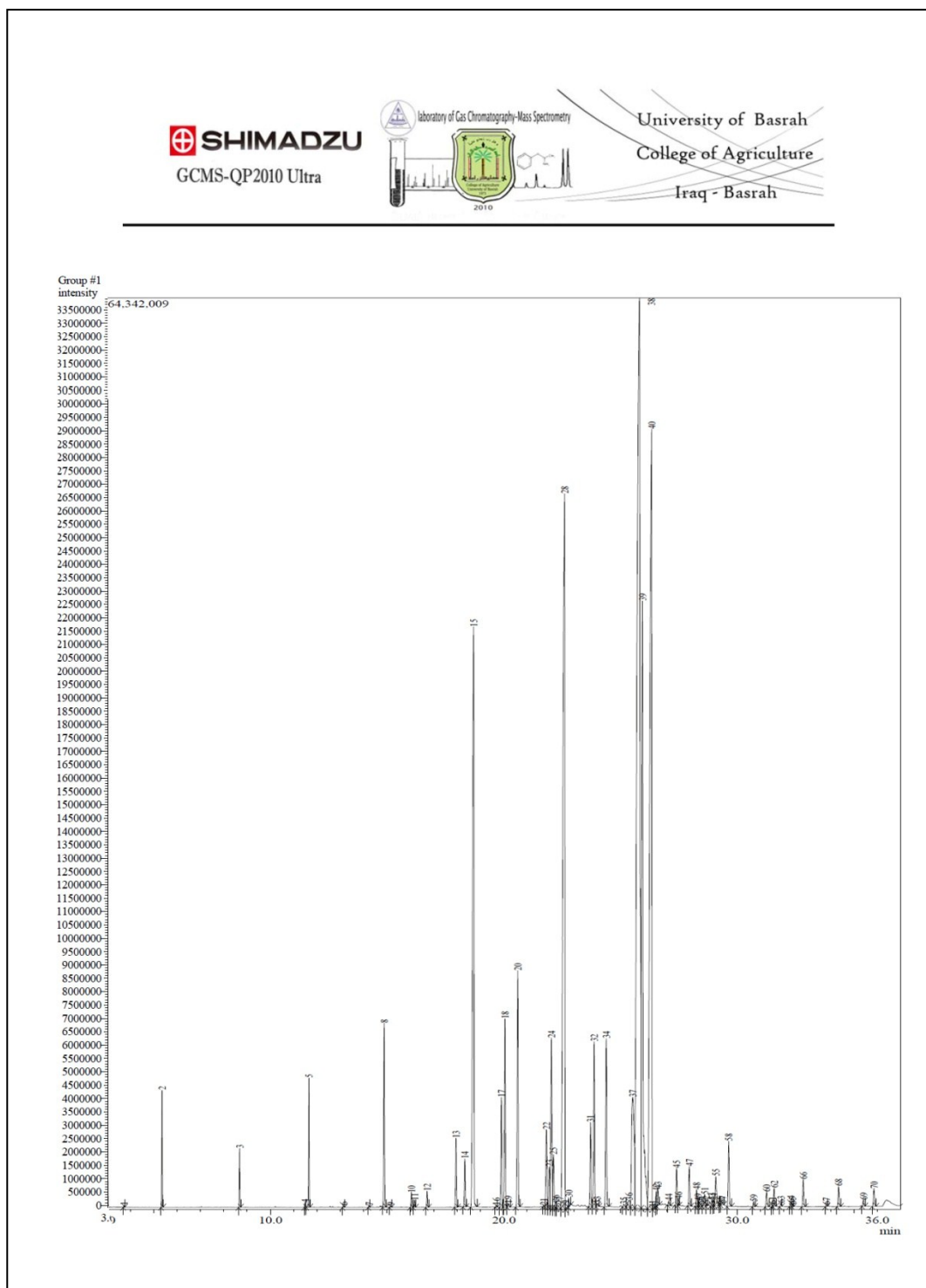
شكل ( 3 ) يوضح مرتسم تحليل الأحماض الدهنية في حليب الجاموس بواسطة جهاز الـ ( GC-MS )
