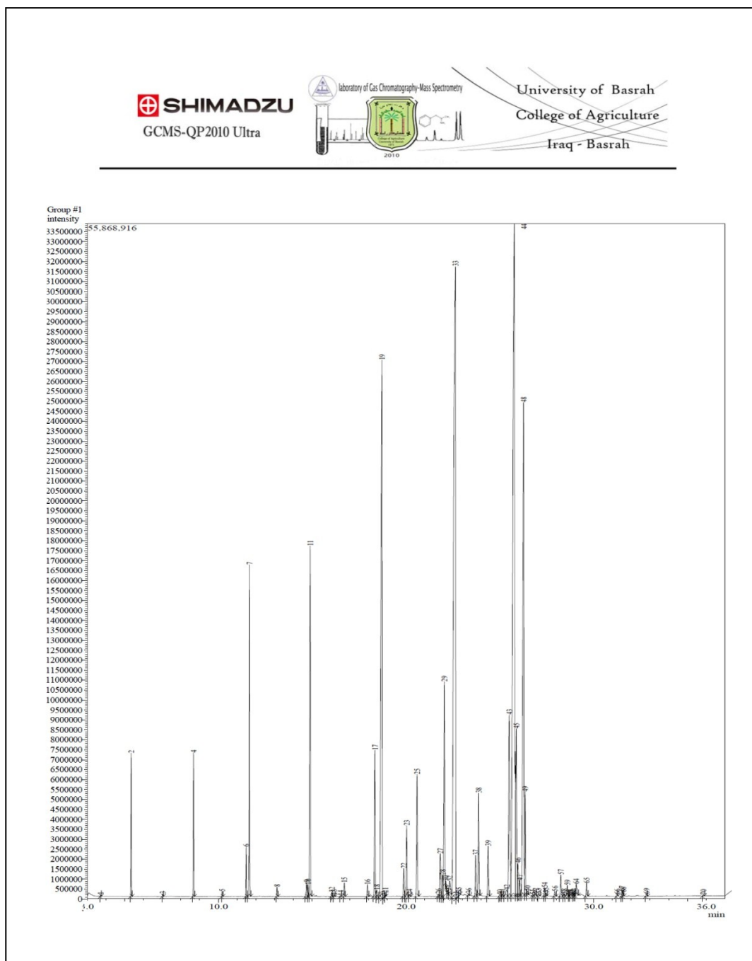
شكل ( 2 ) يوضح مرتسم تحليل الأحماض الدهنية في حليب الأبقار بواسطة جهاز الـ ( GC-MS )
