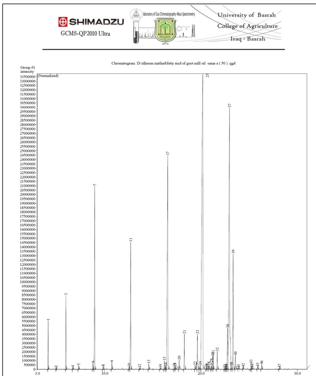
شكل ( 1 ) يوضح مرتسم تحليل الأحماض الدهنية في حليب الماعز بوساطة جهاز الـ ( GC-MS )
