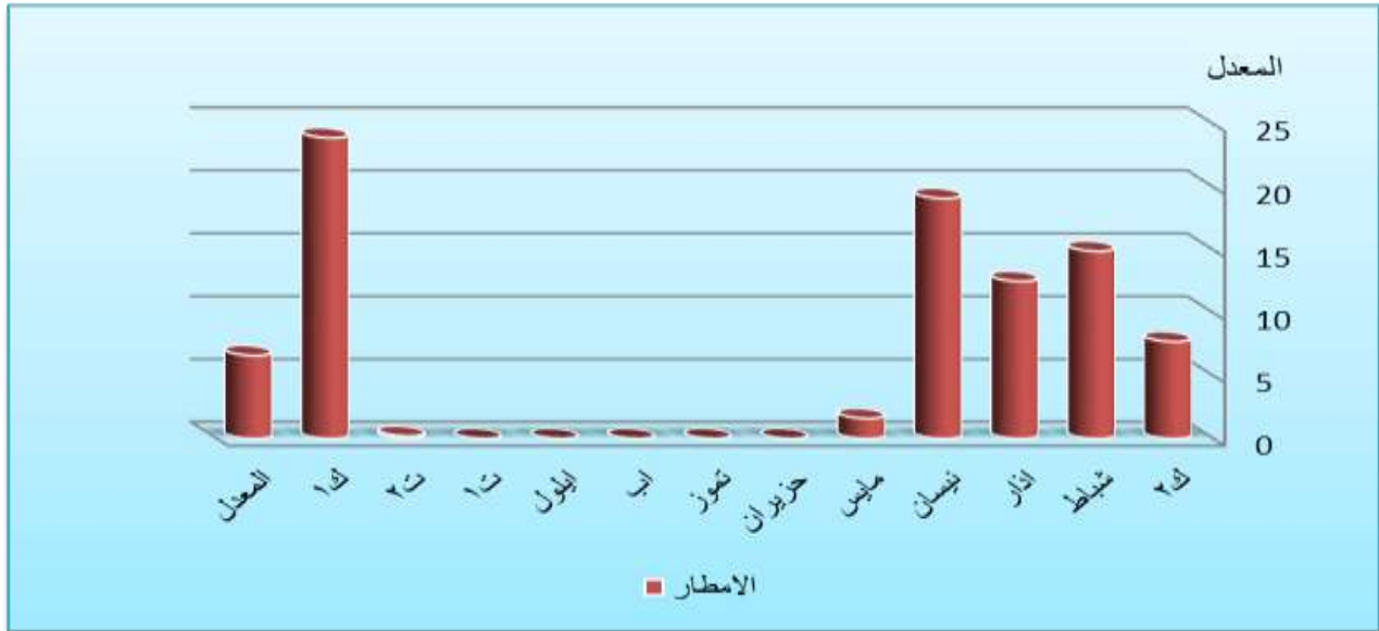
شكل (2) المعدلات الشهرية للأمطار في محطة البرجسية لسنة 2016
