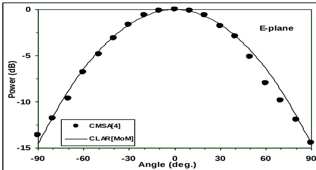
شكل (4) مقارنة الهياكل الإشعاعية للهوائي الشريطي الدائري المحمل بحلقة معدنية و الهوائي الشريطي الدائري عندما ينتشر بدخلة النمط TM_{11} .
