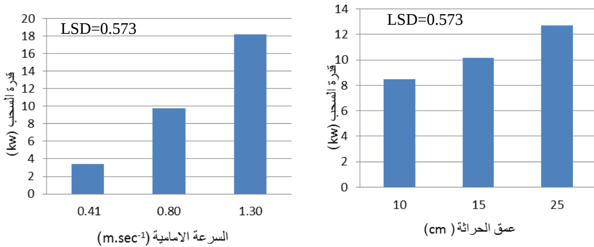
شكل (3) : تأثير عمق الحراثة على قدرة السحب
