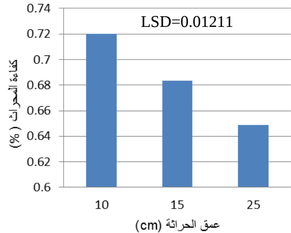
شكل (9) : تأثير عمق الحراثة على كفاءة المحراث
