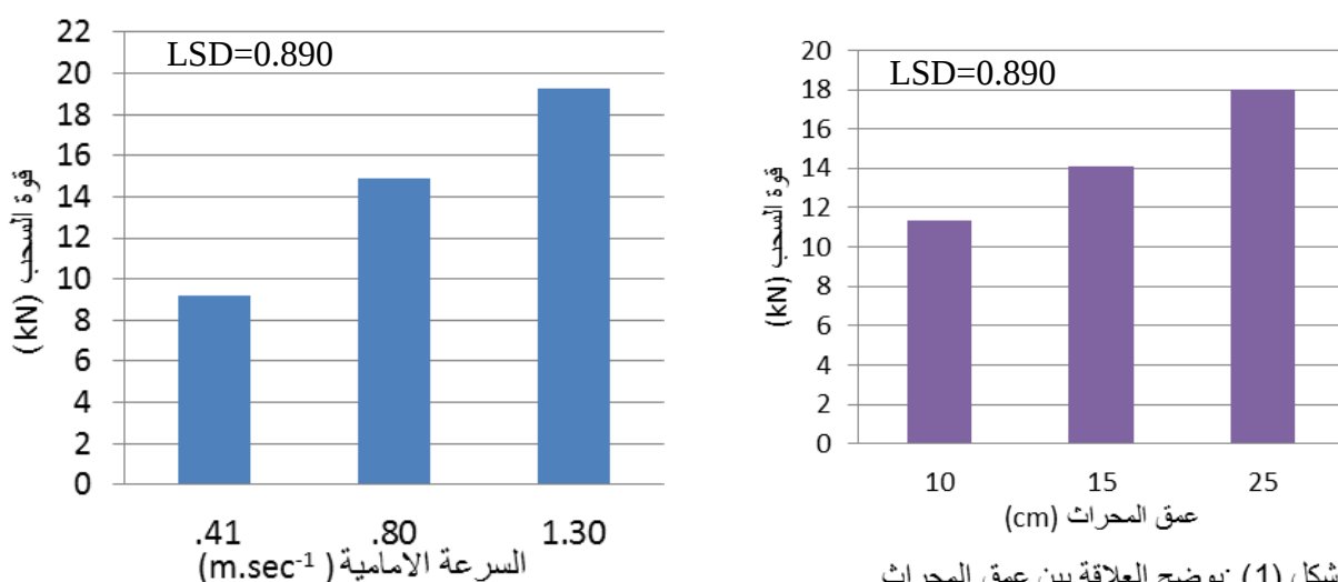
شكل (2) : يوضح العلاقة بين السرعة الامامية وقوة السحب
