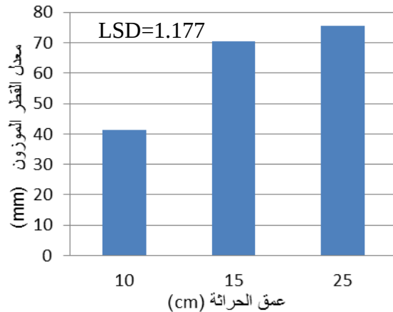
شكل (7) : تأثير عمق الحراثة على معدل القطر الموزون
