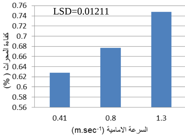
شكل (10) : تأثير السرعة الامامية على كفاءة المحراث
