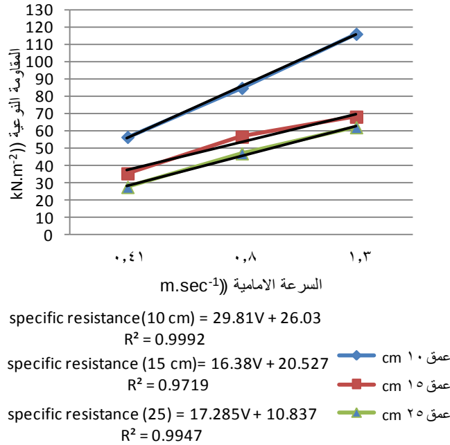
شكل (١٥) : تأثير التداخل بين السرعة الامامية والعمق على المقاومة النوعية
