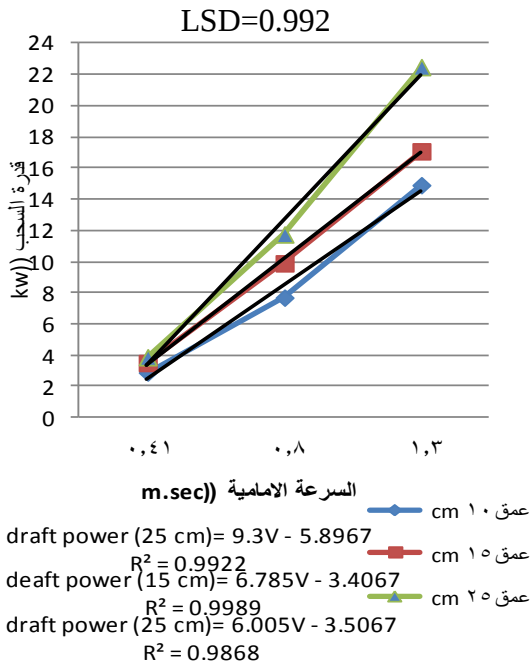
شكل (١٤) : تأثير التداخل بين السرعة الامامية والعمق على قدرة السحب
