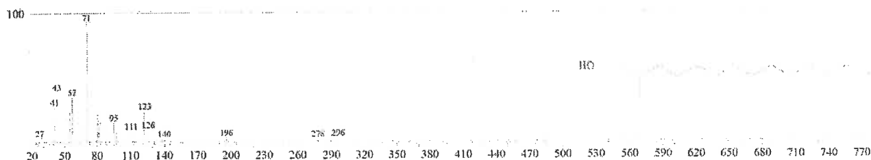
Phytol
