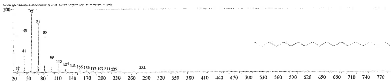
Eicosane
