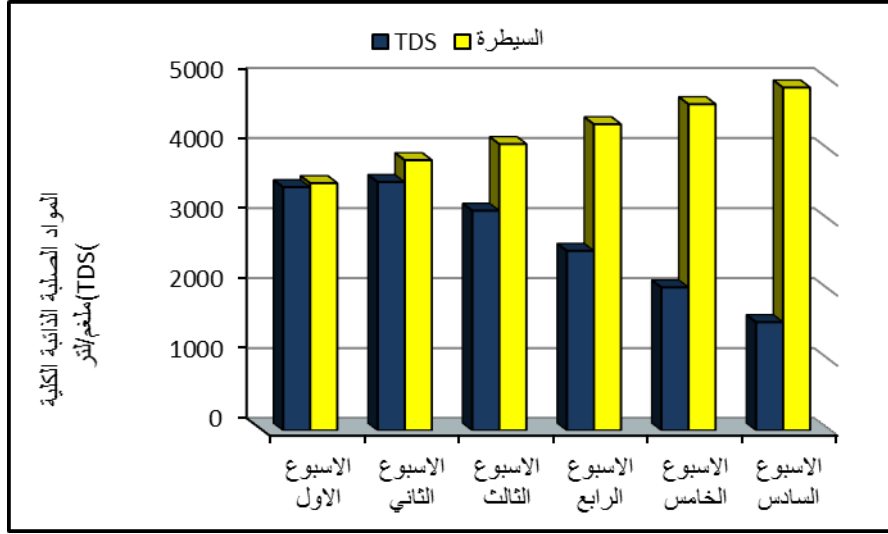
شكل (4) معدل انخفاض المواد الصلبة الذائبة الكلية (TDS) في أحواض المعالجة بنباتات القصب P. australis
