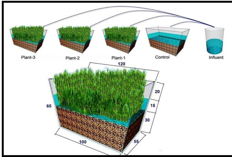
شكل (1) منظومة المعالجة النباتية بأسطح الجريان الحرة (FWS) باستخدام نبات القصب P. australis (تم الرسم ببرنامج 3Dmax)
