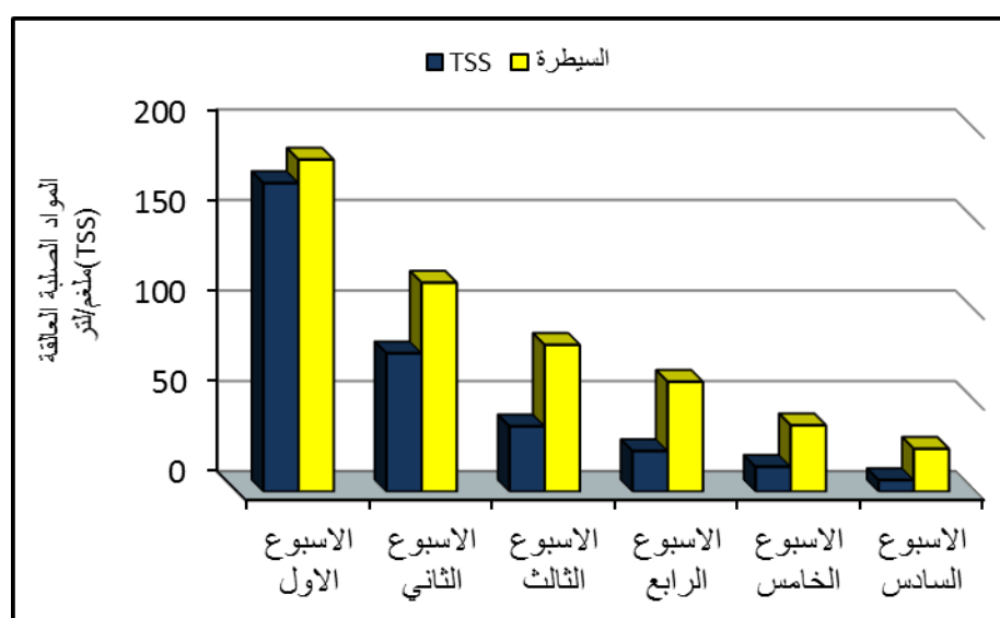
شكل (3) معدل انخفاض المواد الصلبة العالقة الكلية (TSS) في أحواض المعالجة
