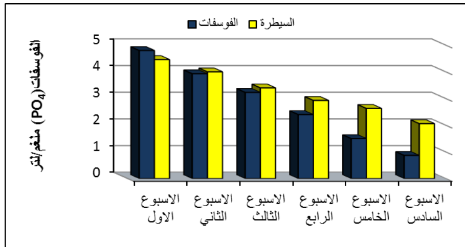
شكل (8) معدل انخفاض الفوسفات ( \text{PO}_4 ) في أحواض المعالجة
