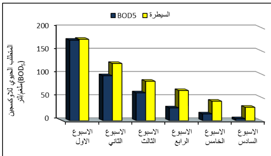
شكل (5) معدل انخفاض المتطلب الحيوي للأوكسجين ( BOD_5 ) في أحواض المعالجة بنباتات القصب P. australis
