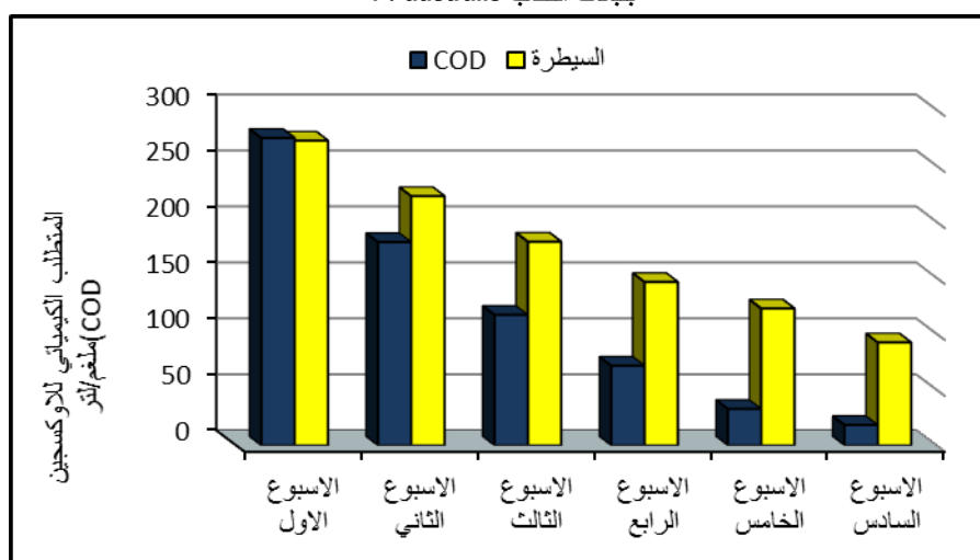
شكل (6) معدل انخفاض المتطلب الكيميائي للأوكسجين (COD) في أحواض المعالجة بنباتات القصب P. australis
