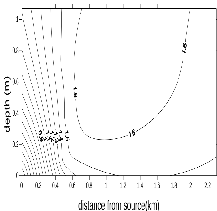
(شكل ١١) توزيع B. D مع العمق والمسافة عن مصدر الترسيب في المسار الثاني
